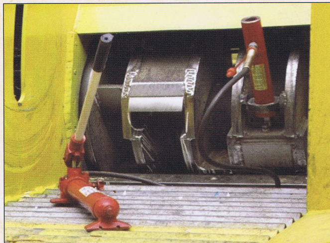
Messer-Schnellwechselsystem
